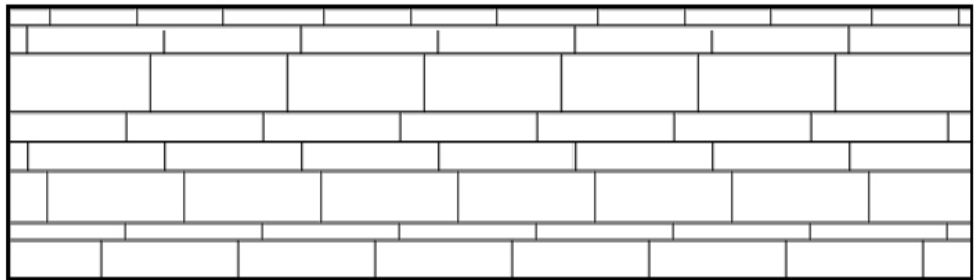
Parquet à la française (à joints perdus)
